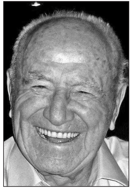
Efel
